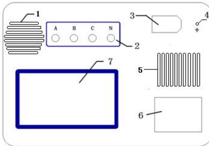
图 5.1 面板图
