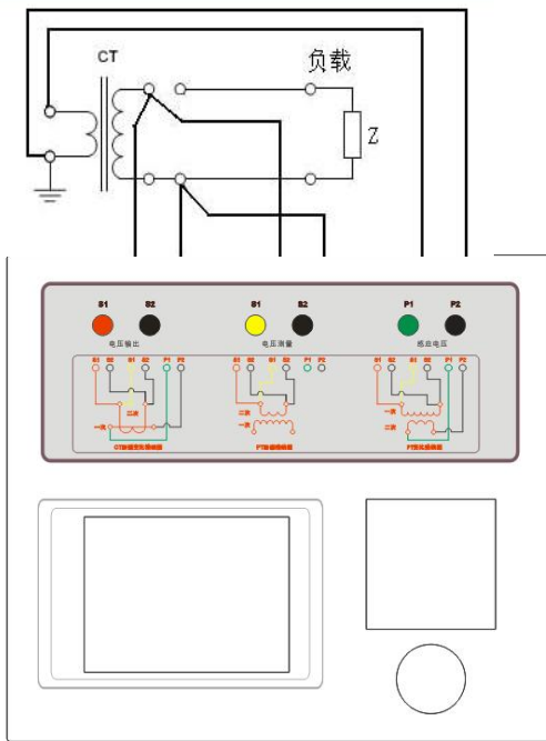
图 2.1 CT 直阻、励磁、变比试验接线方式
