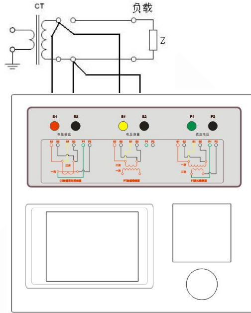
图 2.2 CT 二次负荷试验接线方式
