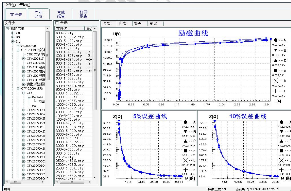
图 3.7 多个文件合并转换时曲线界面
