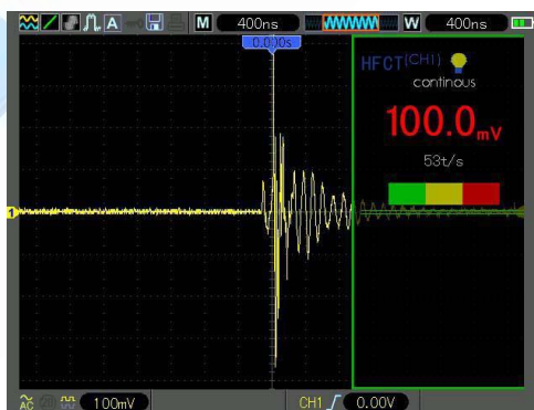
传感器饱和
