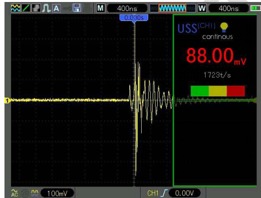
传感器饱和
