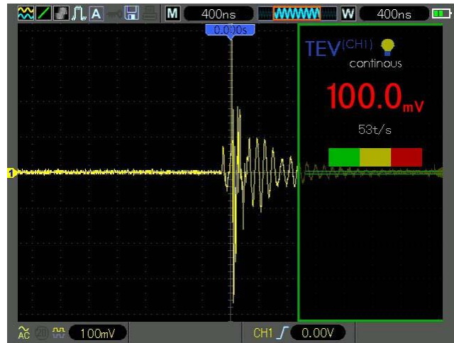
传感器饱和
